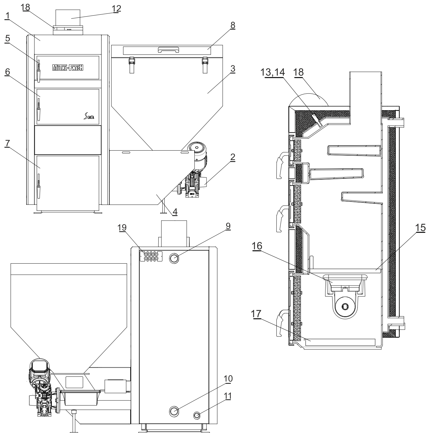
Рисунок 7.1 Основные элементы конструкции котла SMART и SMART EKO
