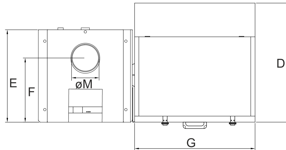
Рисунок 7.2.1 Размеры котла SMART
