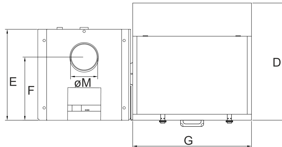
Рисунок 7.3.1 Размеры котла SMART EKO
