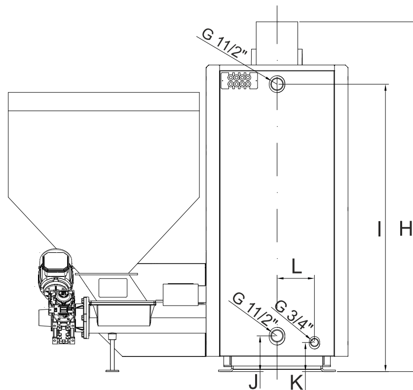
Рисунок 7.2.1 Размеры котла SMART
