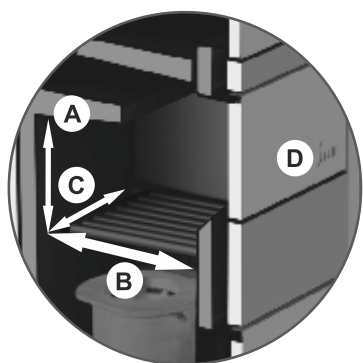
Рисунок 7.2.2 Размеры запасной топочной камеры и загрузочного отверстия SMART
