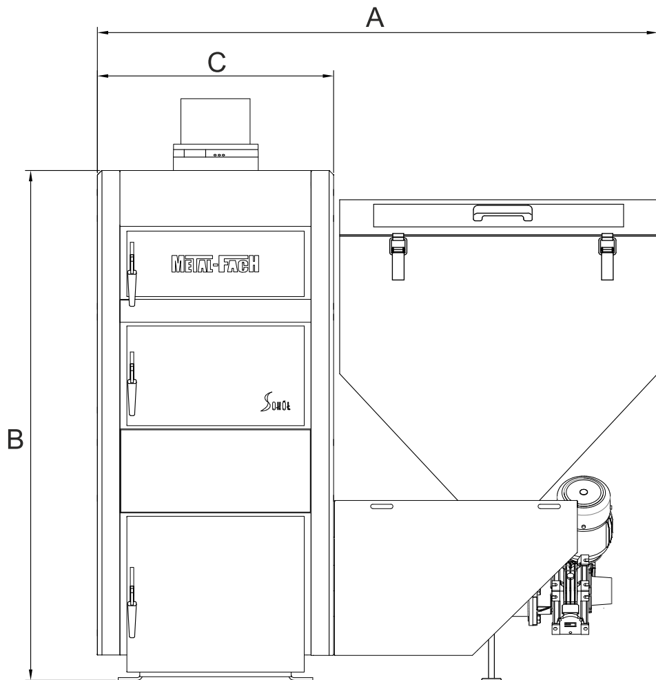
Рисунок 7.2.1 Размеры котла SMART
