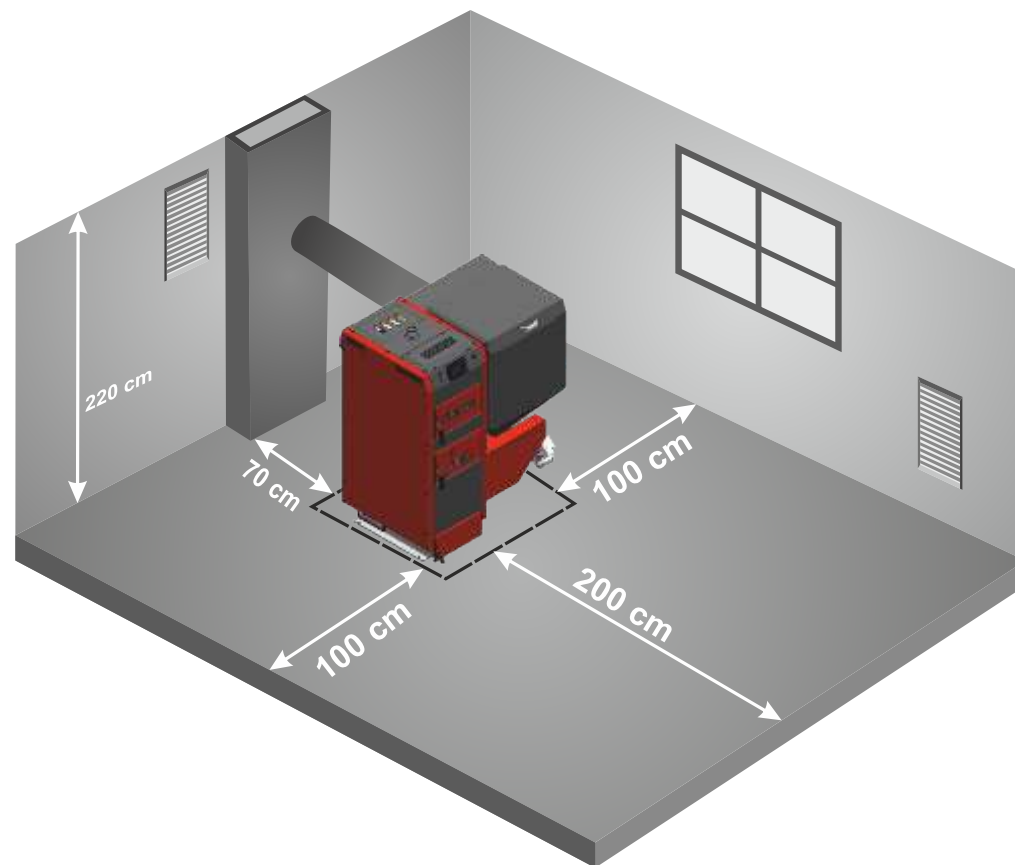
Рисунок 8.1 Минимальные расстояния при установке котла в котельной
