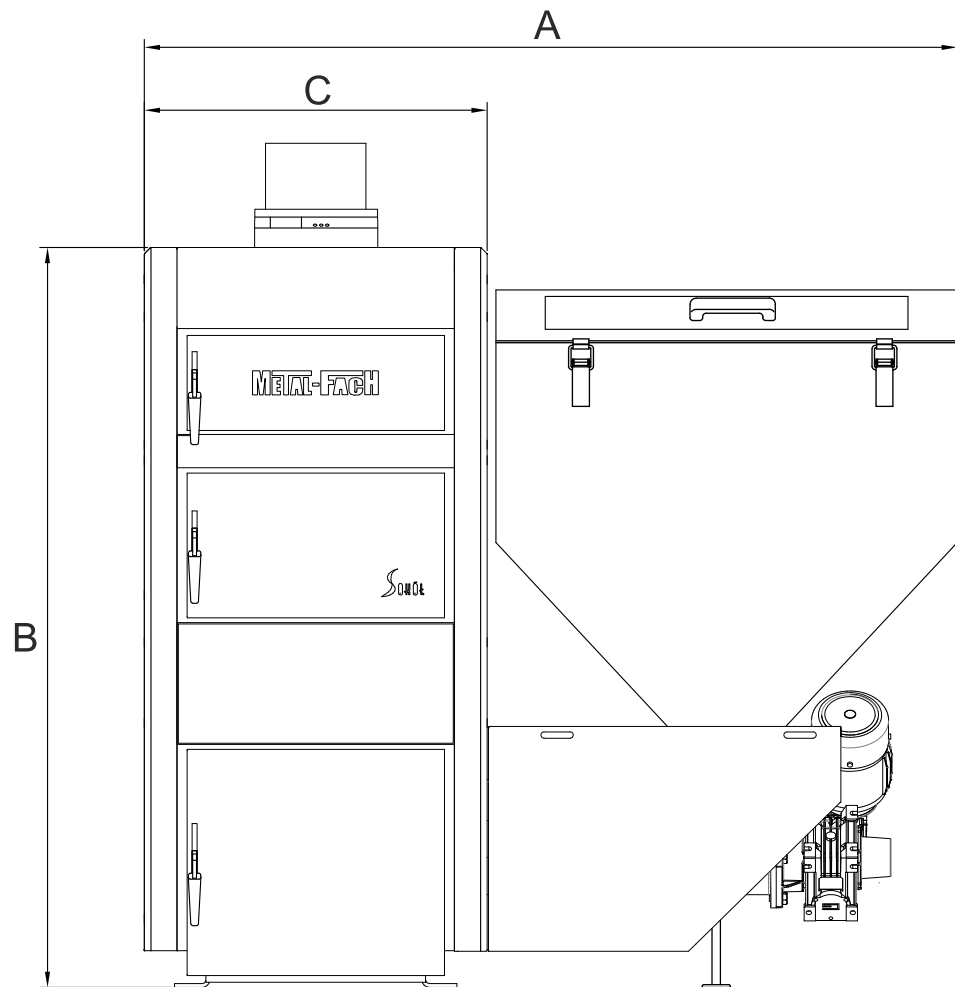
Рисунок 7.3.1 Размеры котла SMART EKO
