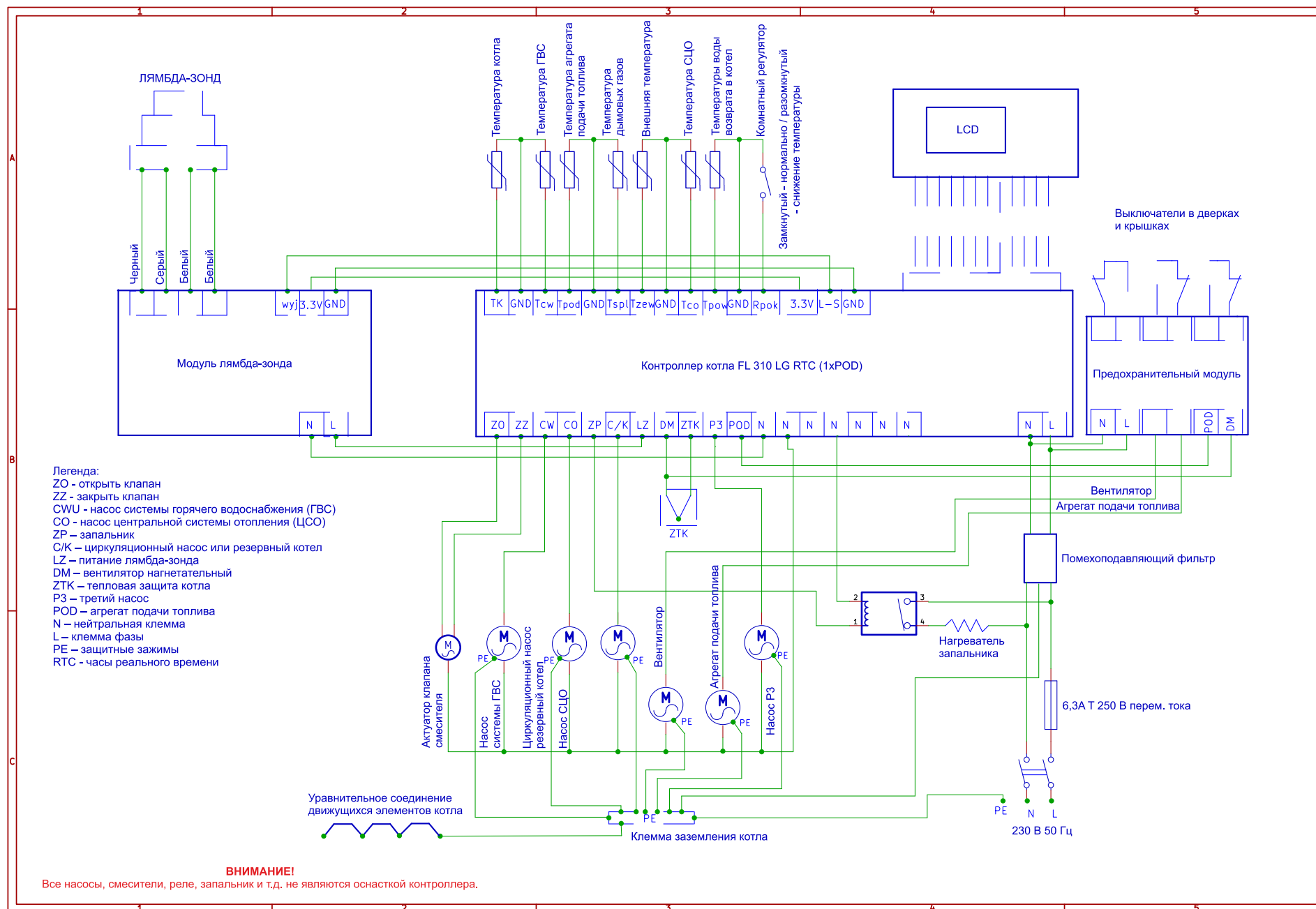
Рисунок 10.1 Электрическая схема подключения котла
