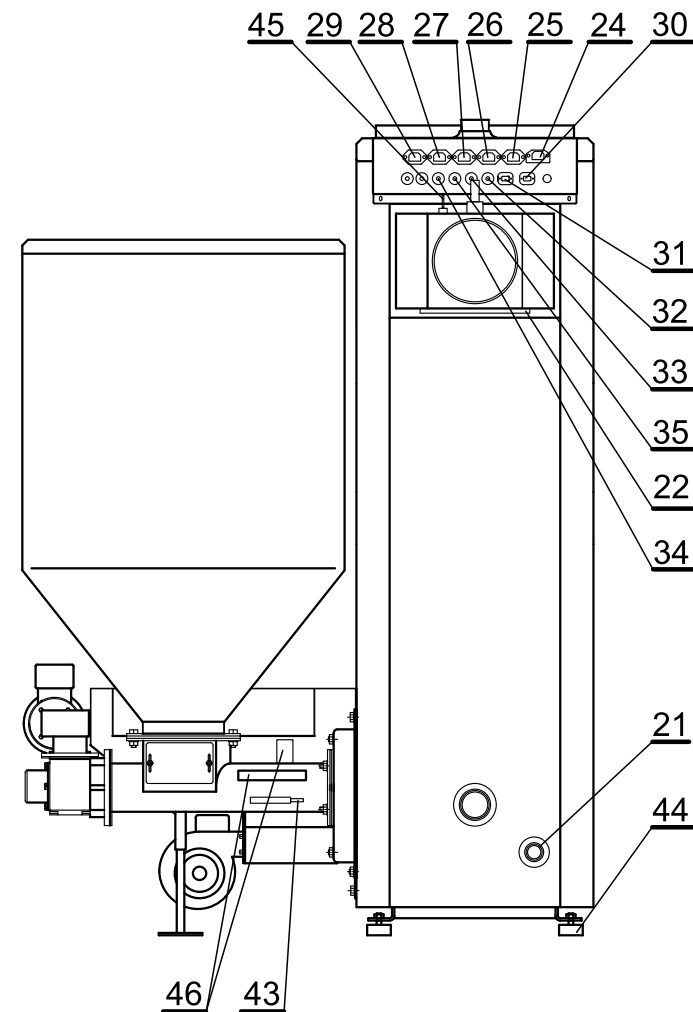
Рисунок 7.1 Основные элементы конструкции котла SD DUO и SD DUO BIO
